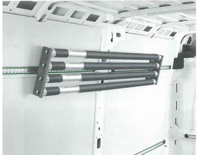
12 + 13 Ungesicherte Ladung stellt für Mensch und Material eine Gefahr dar. Mit Spannnetzen oder Spannstangen kann das Material zügig und langanhaltend gesichert werden. Fotos: Bott
